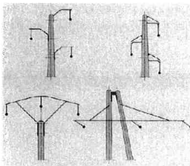
Figure 4 : Réseau électrique HTA nu - Technique suspendue
